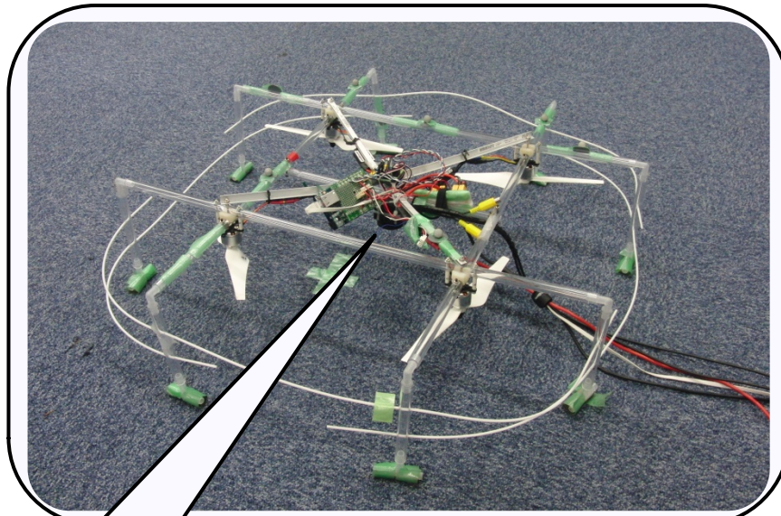
検査ヘリコプター
